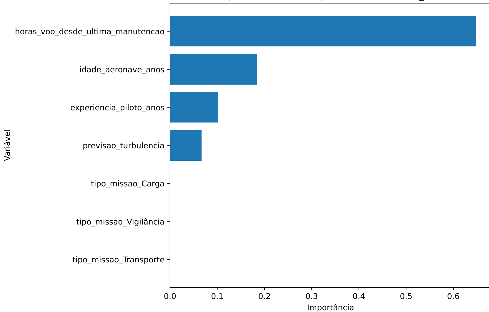
Top variáveis mais importantes — decision_tree
